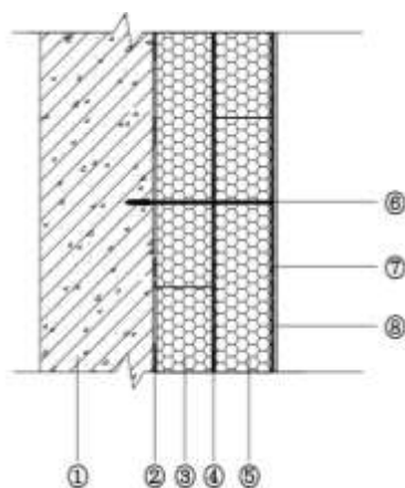
图 C. 0. 2 双层保温板外保温系统基本构造
